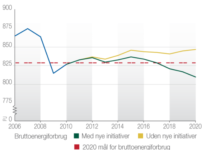
Figur 5: Udviklingen i bruttoenergiforbruget i Danmark 2006-20
