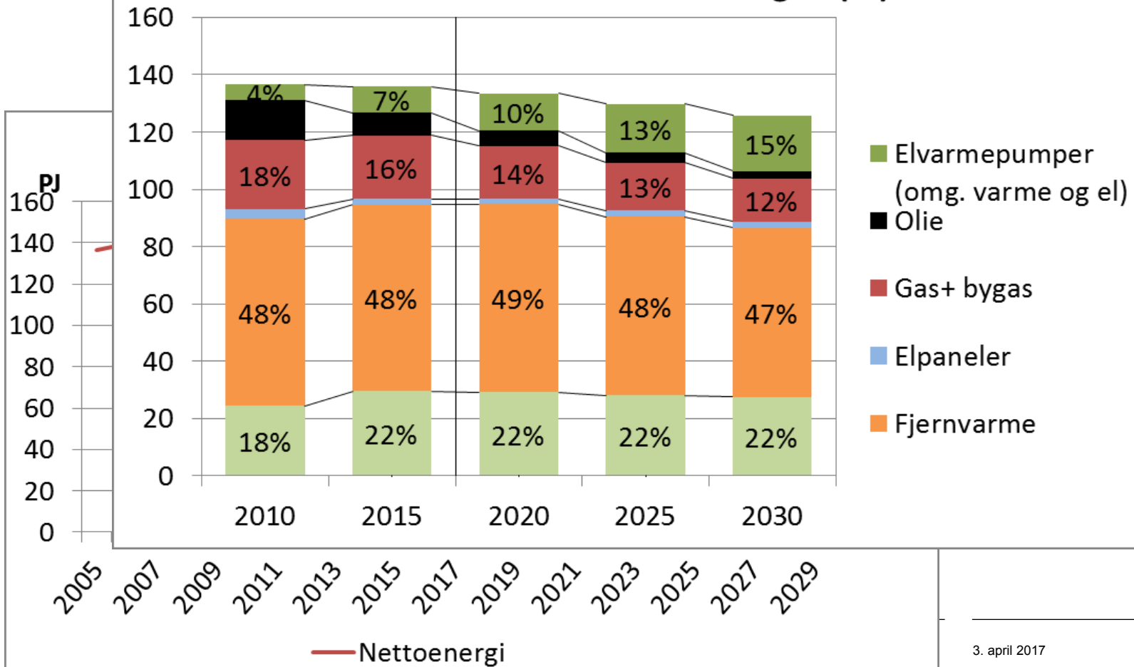
Nettovarmebehov fordelt teknologier (PJ)
