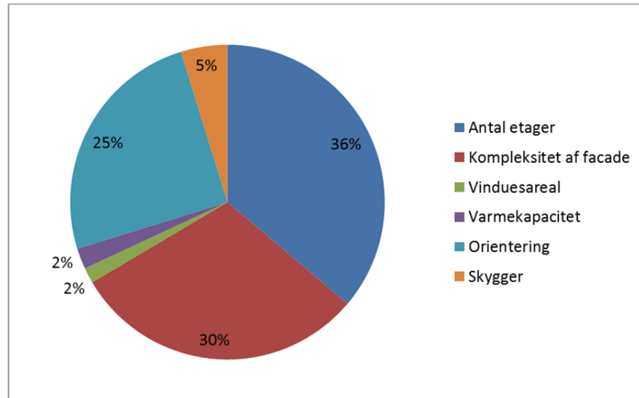
Figur 5. Betydningen af enkeltparametre fra modellen med højest energibehov til modellen med lavest energibehov.
