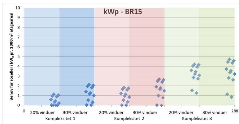
Figur A.7. Antal etager 6.
