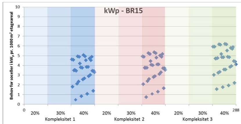
Figur B.10. Vinduesareal 40 %.
