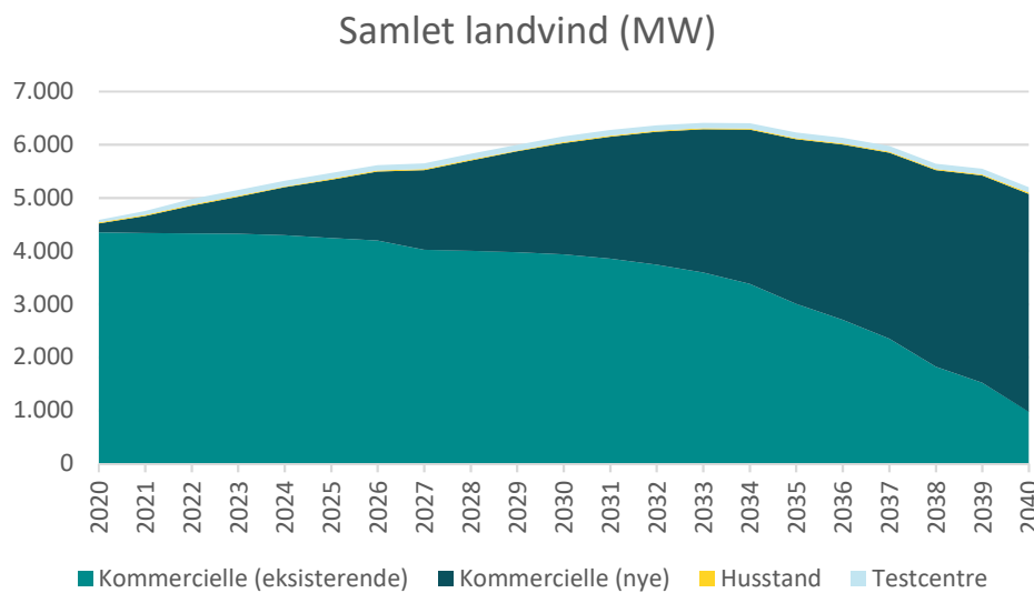
Figur 1: Samlet landvind i AF20 (MW).
