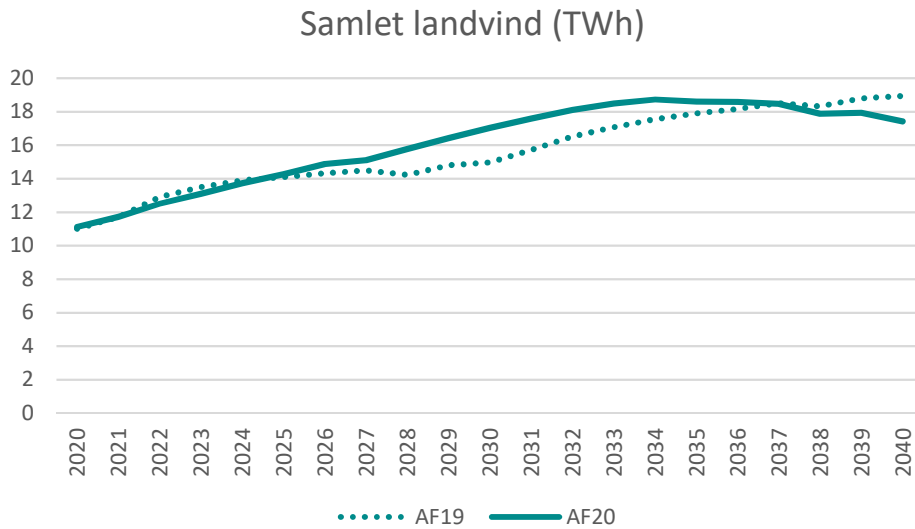
Figur 4: Samlet produktion fra landvind i AF19 og AF20 (TWh).
