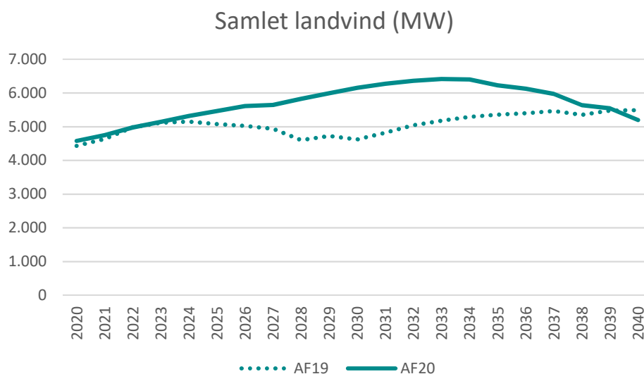
Figur 3: Samlet landvind i AF19 og AF20 (MW).
